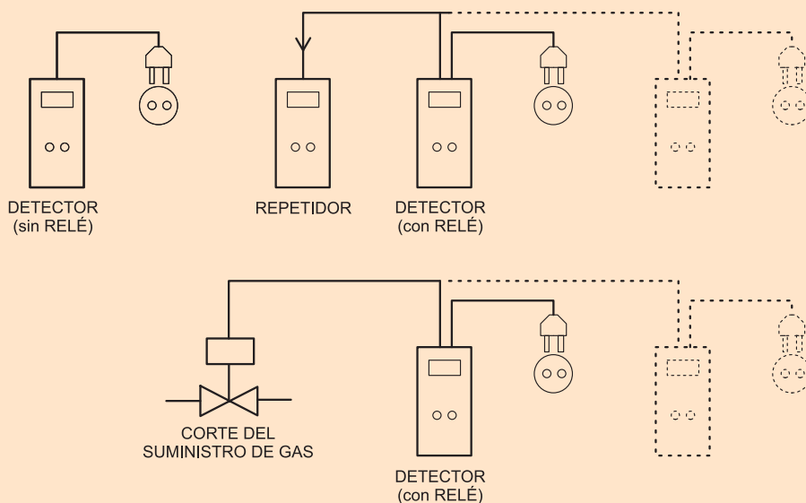
CONEXIONADO CON UNIDAD REPETIDORA
