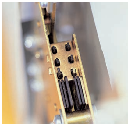
Cerradura de gorjas de alta seguridad.
